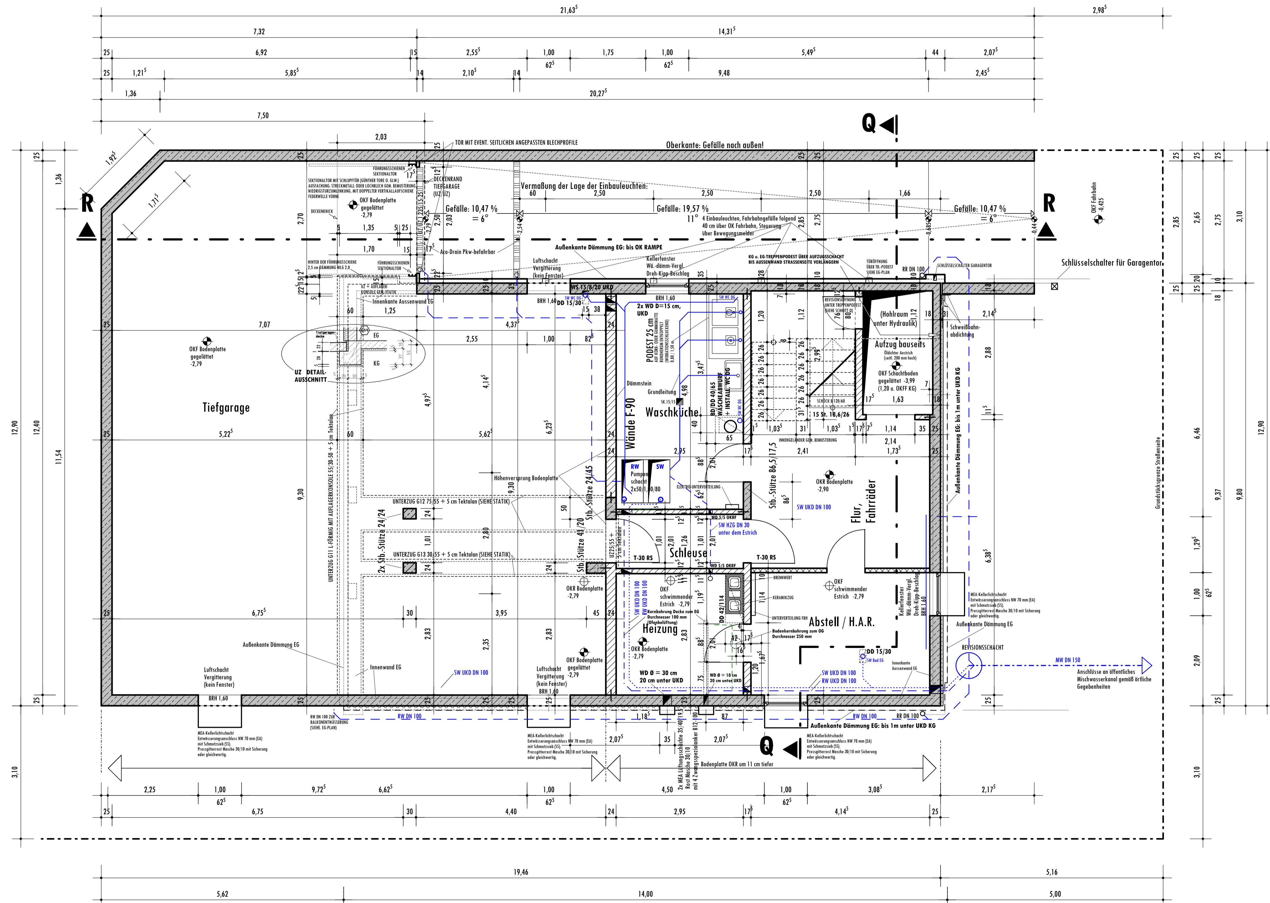
KELLERGESCHOSS Alle Innentüren mit breiten Türhähnen Alle Fenster in grau RAL 7040
