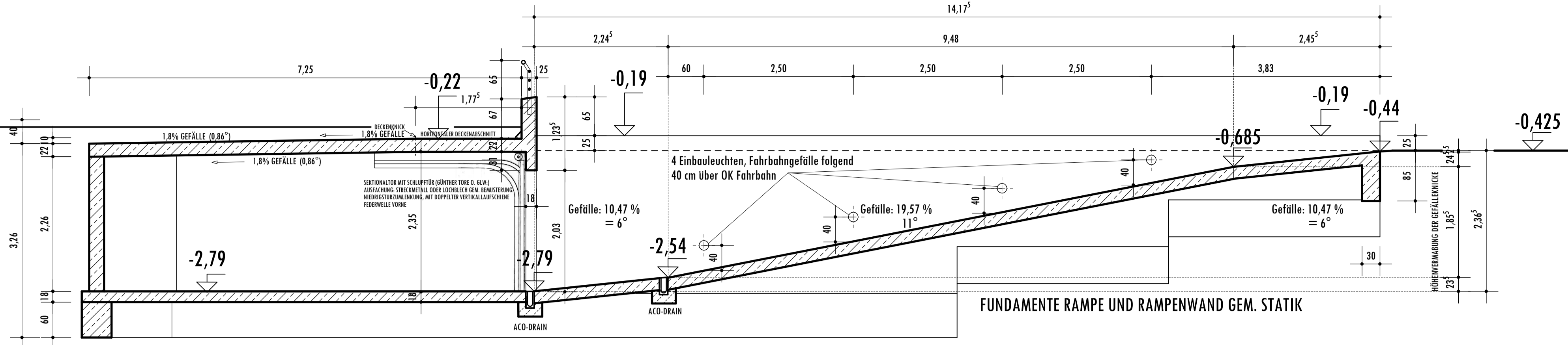
SCHNITT R (RAMPE)
